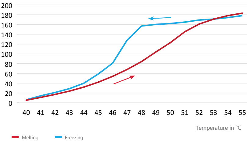
Enthalpy (J/g)
