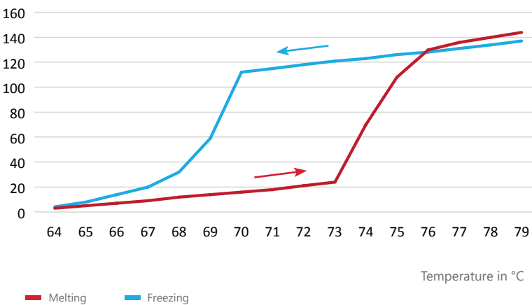
Enthalpy (J/g)
